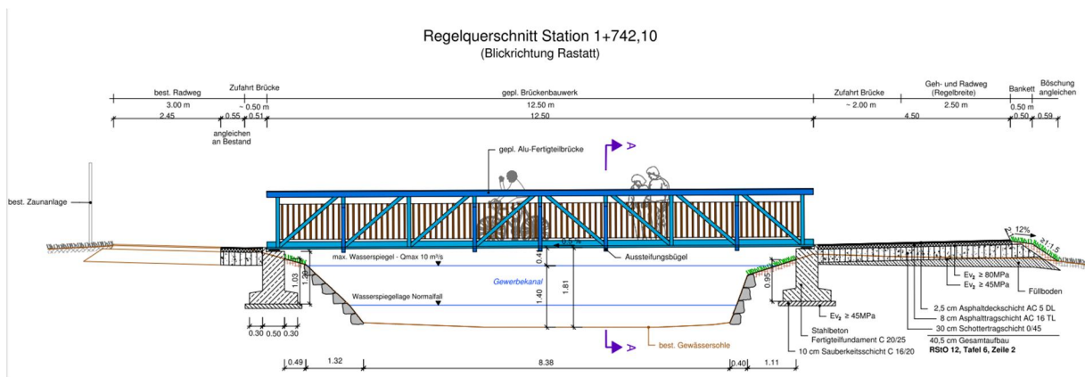
Regelquerschnitt geplantes Brückenbauwerk über den Gewerbekanal
