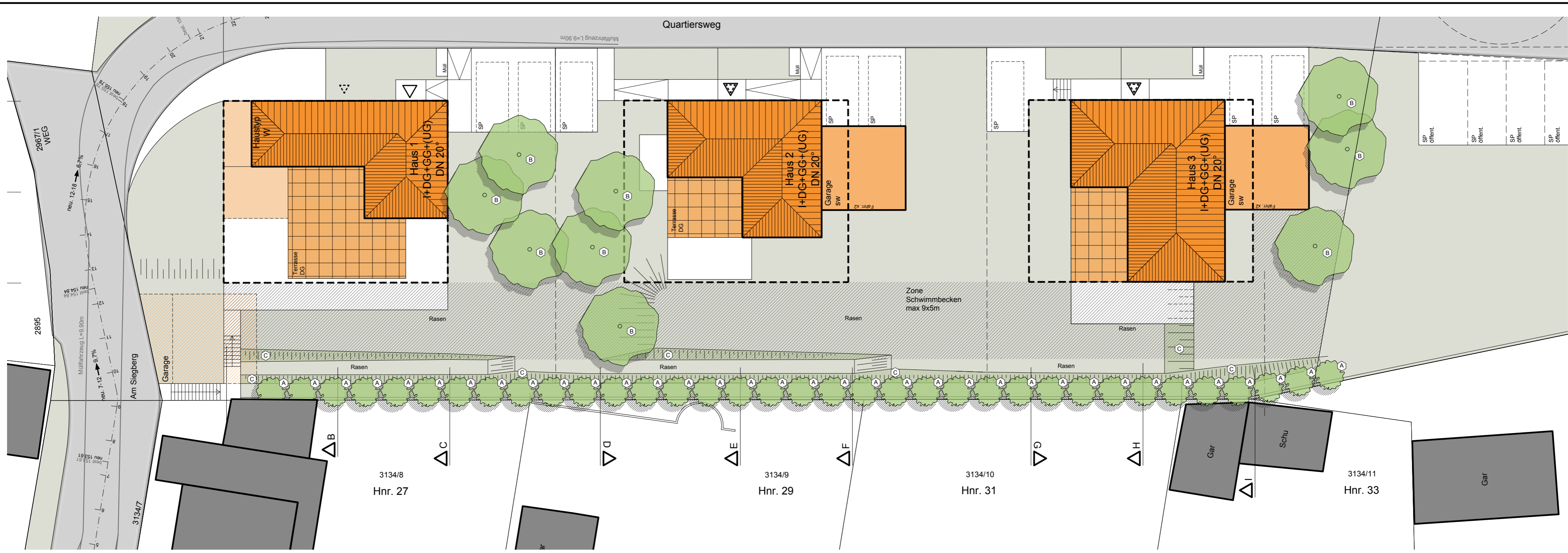
Landschaftsbau Lageplan
